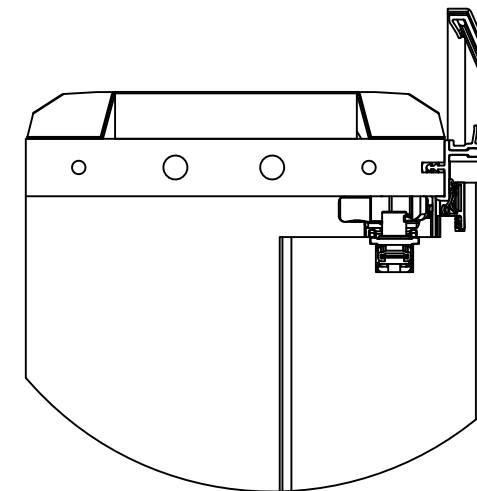
DETAIL Z 2 : 5
