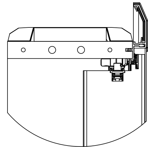
DETAIL Z 2 : 5
